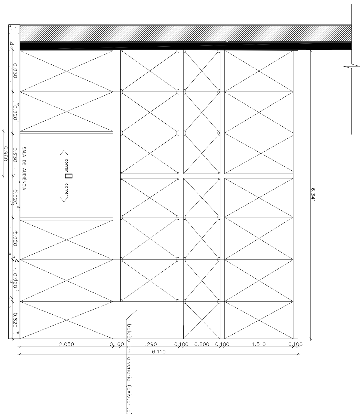
VISTA FRONTAL ESQUADRIA – SITUAÇÃO ATUAL
