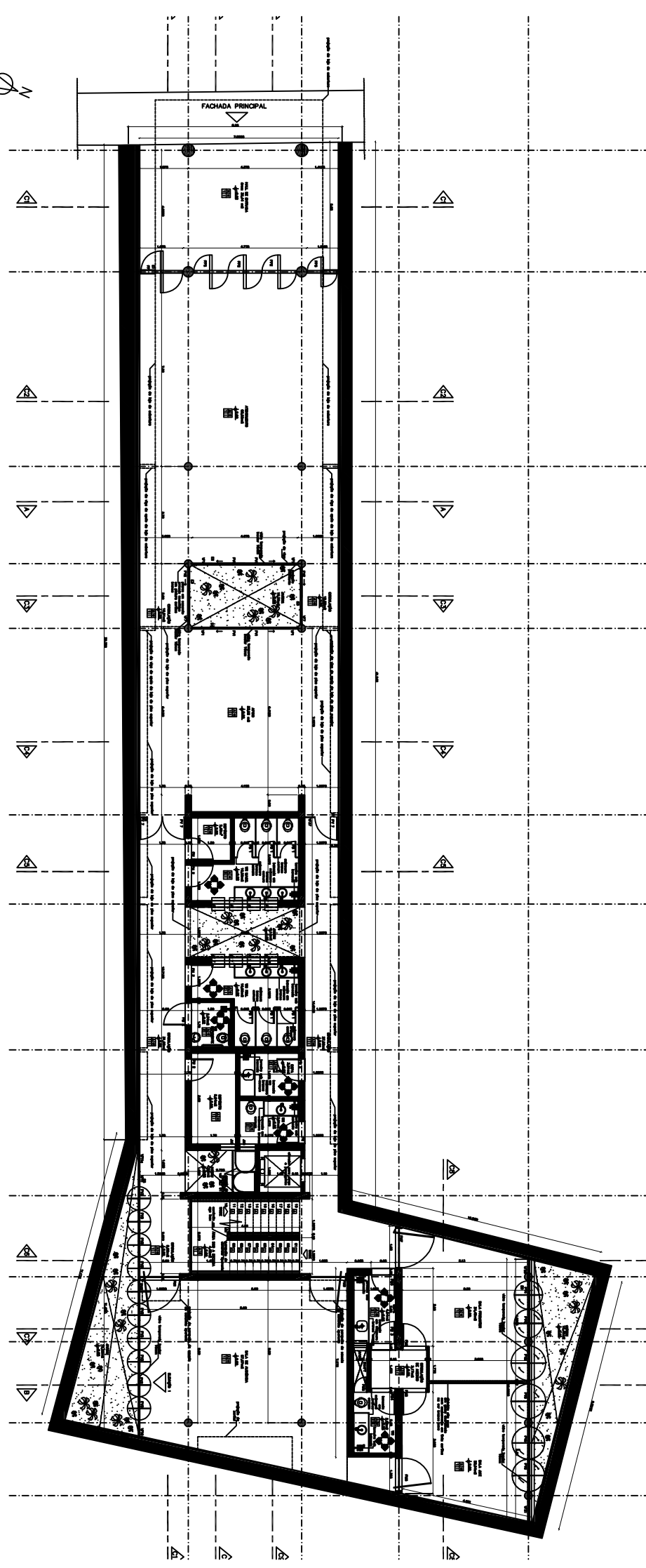
PLANTA BAIXA PAVIMENTO TERRECO ESCALA 1:50
