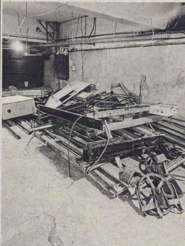
Foto 02: PEÇAS METÁLICAS DO ELEVADOR DESMONTADO
